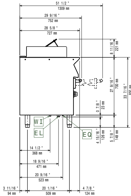
Oldalnézet
